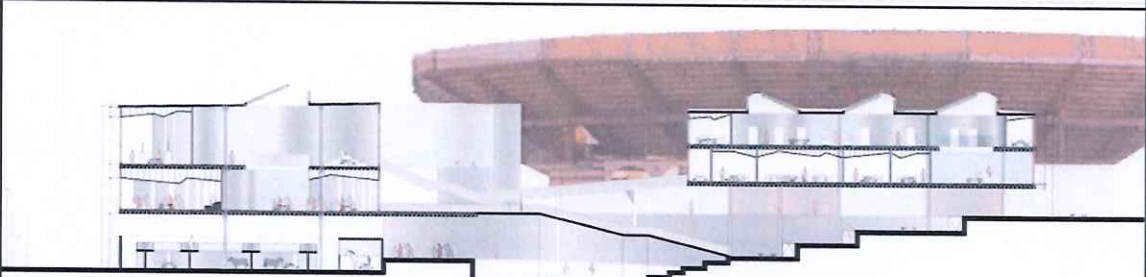
SECCION A-A 1/150
