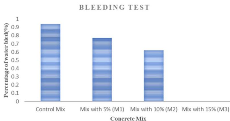
Fig. 8 - Mix Bleed
