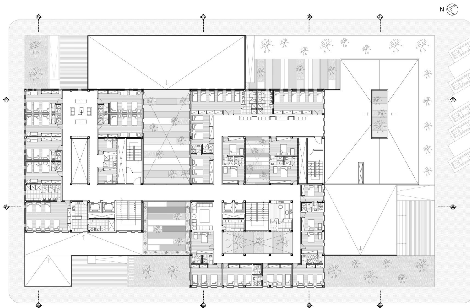
Ilustración 79: Planta de distribución – Tercer Nivel. Fuente: Elaboración propia.
