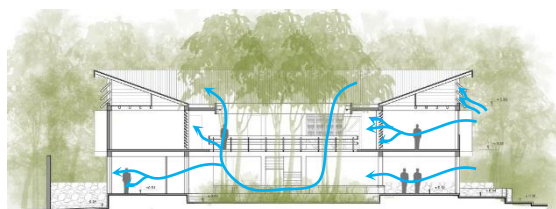
Ventilación cruzada
