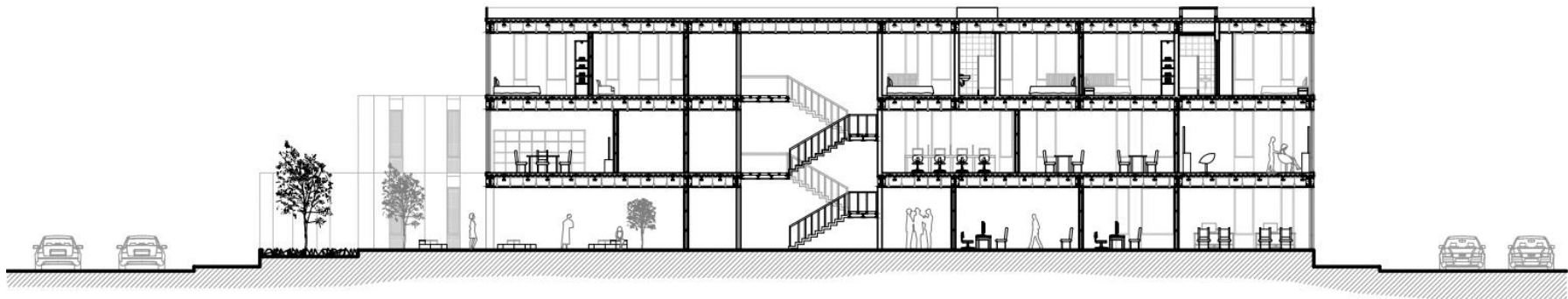
Ilustración 89: Corte transversal 2. Fuente: Elaboración propia.
