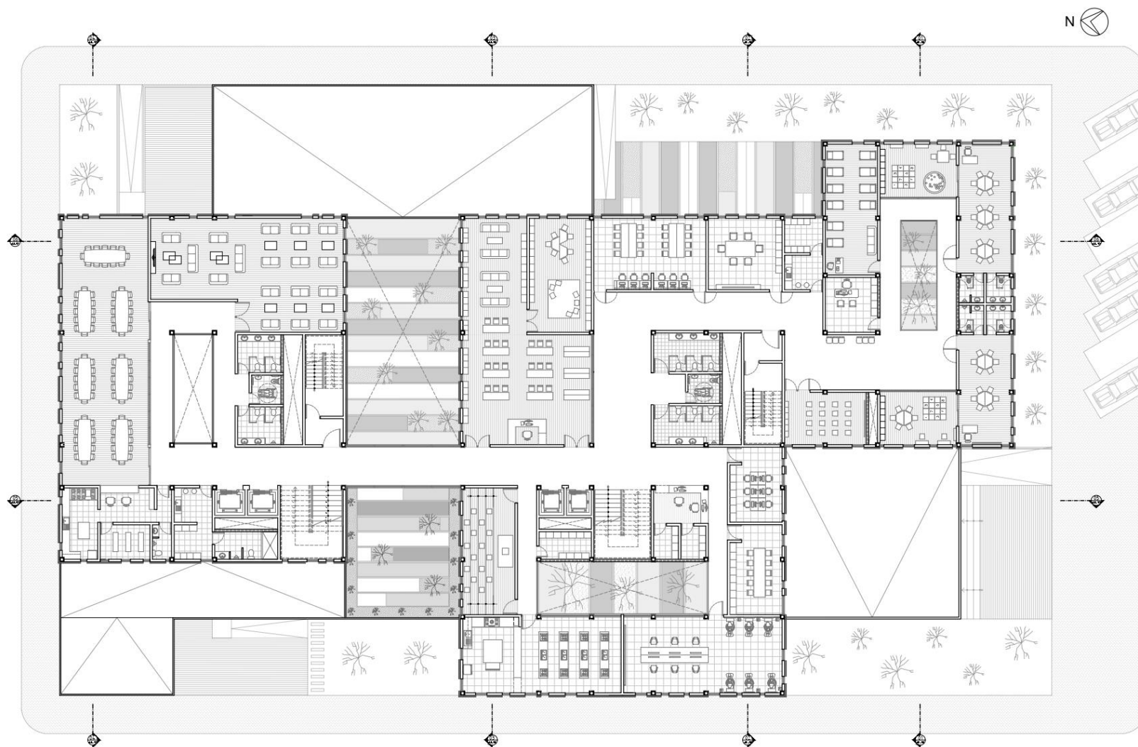
Ilustración 78: Planta de distribución – Segundo Nivel. Fuente: Elaboración propia.
