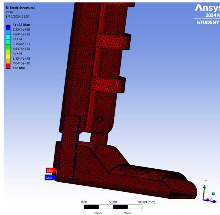
Figura 90: Vida del análisis de fatiga con una fuerza de 4209,4 N
