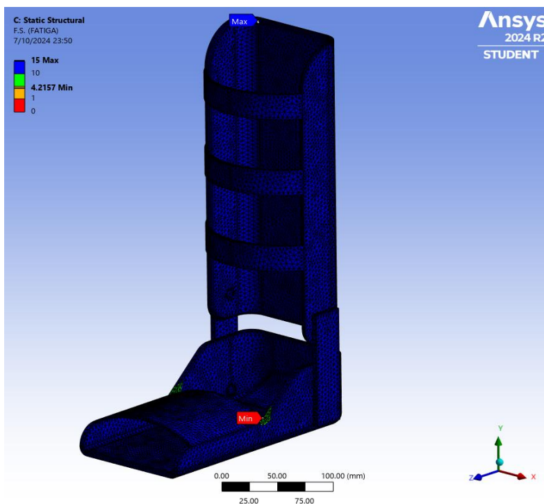
Figura 63: Factor de seguridad mínimo de la órtesis de tobillo y pie (Análisis de fatiga)
